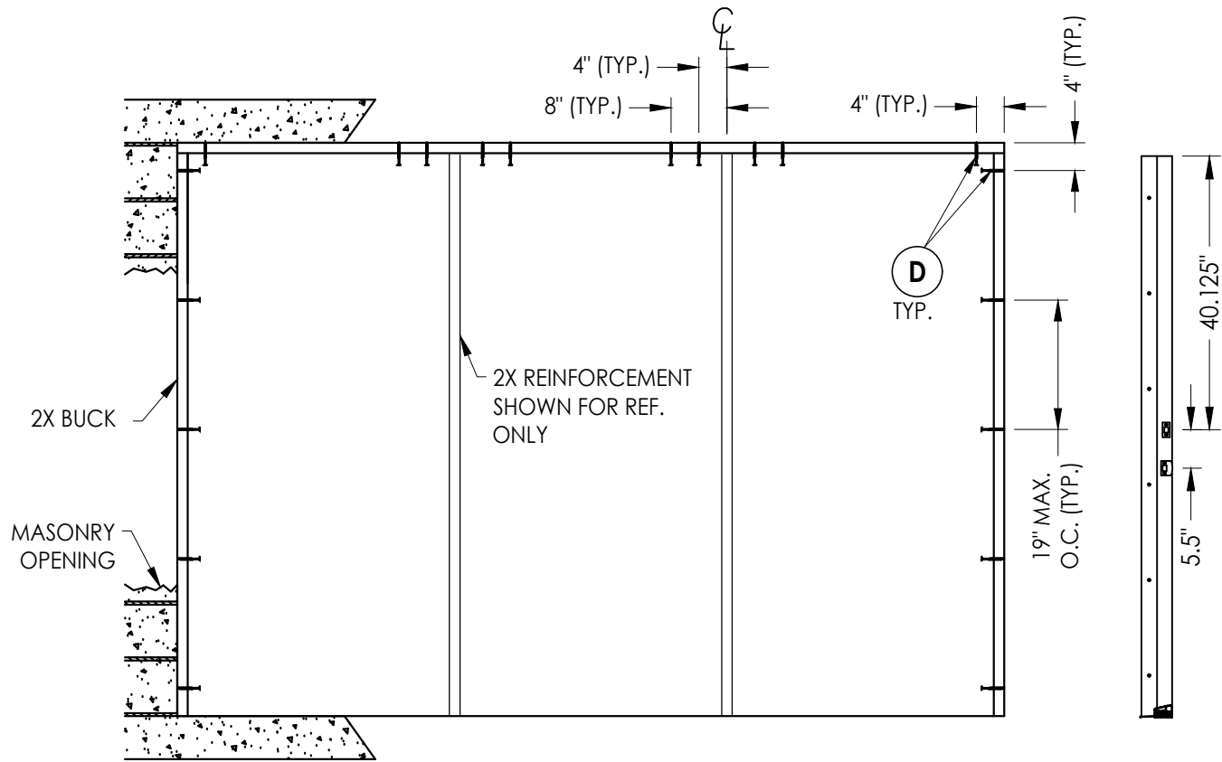
STRIKE JAMB
